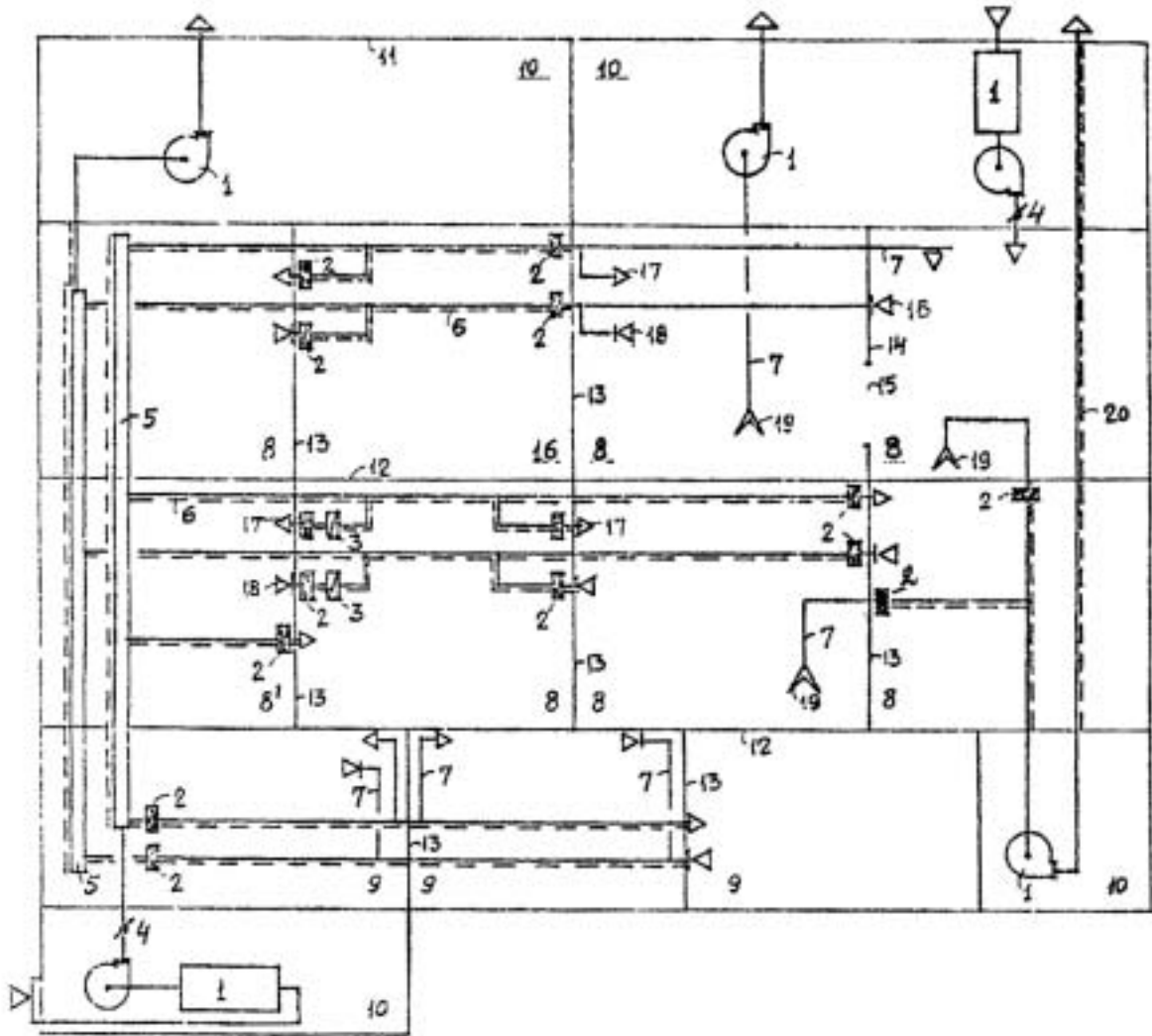
Рис. 3. Схемы воздухопроводов для помещений категории А, Б или В.
