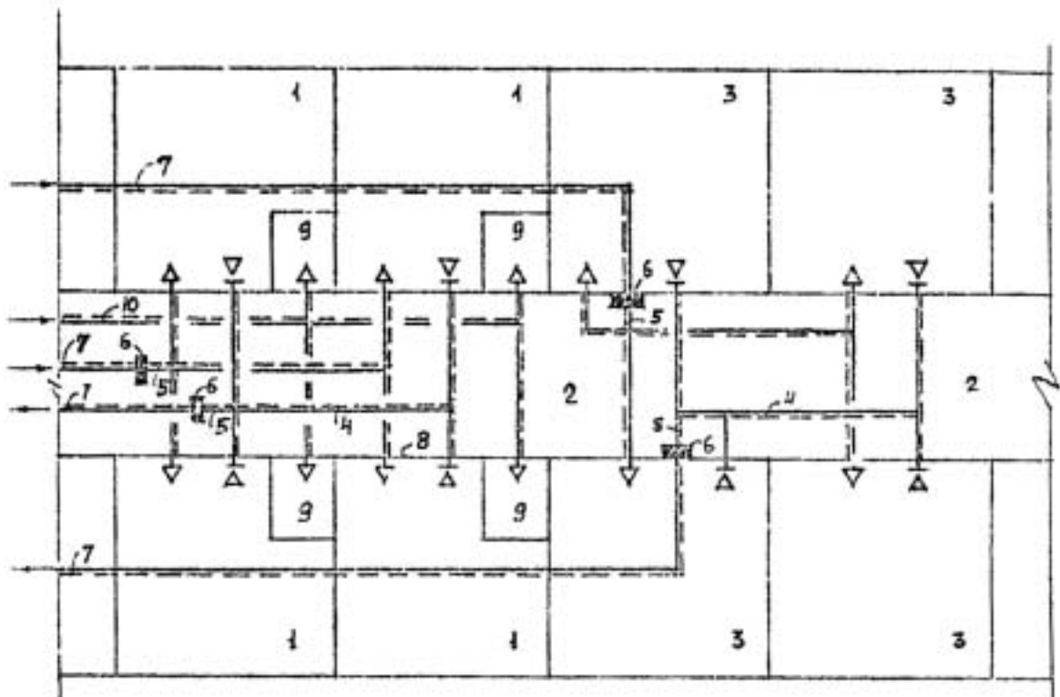
Рис. 6. Схемы воздуховодов для помещений категории А, Б или В с выходами в коридор. 1 - помещения категории А или Б; 2- коридор; 3 - помещение категории В (без тамбуров-шлюзов на выходе); 4 - транзитный сборный воздуховод вытяжной системы с нормируемым пределом огнестойкости по п. 4.118; 5 - участок сборного воздуховода с нормируемым пределом огнестойкости по п. 4.118 длиной не более 1 м от ближайшего к вентилятору ответвления до места установки огнезадерживающего клапана; 6 - огнезадерживающий клапан по п. 4.123 - для помещений категории А и Б в исследовании по п. 4.74; 7 - транзитный воздуховод с пределом огнестойкости по п. 4.118, далее присоединяемый к коллектору или вентилятору; 8 - противопожарная преграда с нормируемым пределом огнестойкости по п. 3.1 СНИП 2.01.02-85*; 9 - тамбур-шлюз для помещений категории А и Б; 10 - транзитный сборный воздуховод с пределом огнестойкости 0,5 часа по п. 4.122 СНИП.
