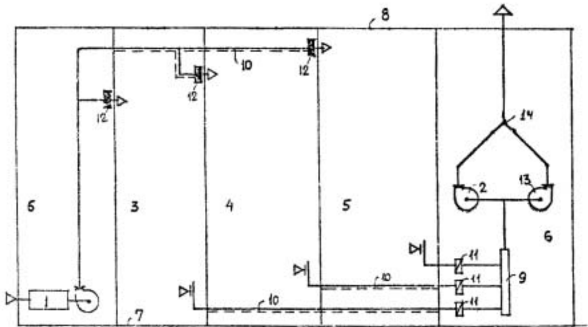
Рис. 5 Схемы воздуховодов для изолированных производственных помещений категорий А, Б или В по п. 4.25 в.
