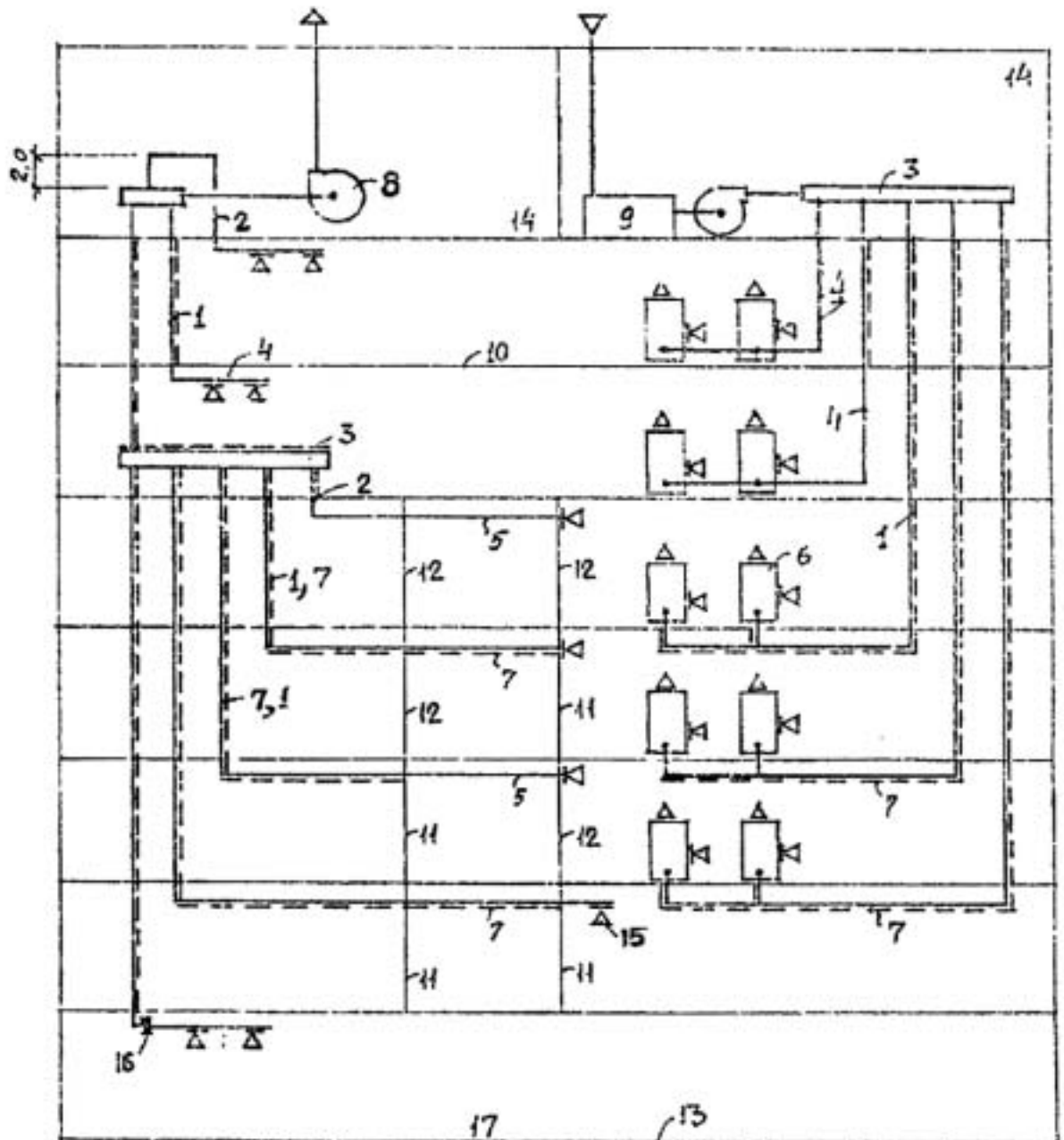
Рис. 2. Схемы воздуховодов с горизонтальными коллекторами.
