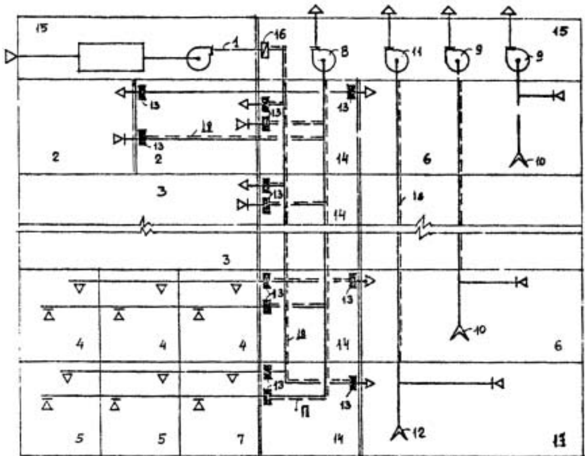
Рис. 7. Схемы воздуховодов для лабораторных помещений.
