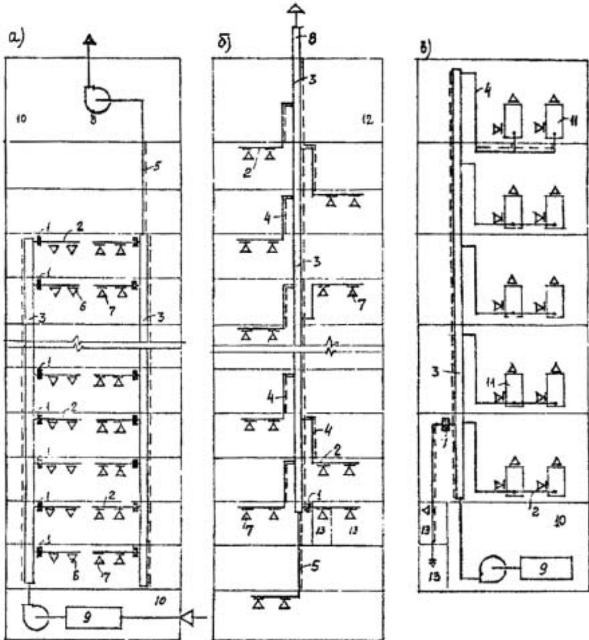
Рис. 1. Схемы воздухопроводов с вертикальными коллекторами.
